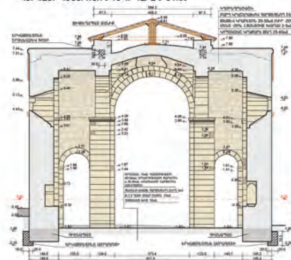
ԿՏՐԱԿԱՆ ԿԵՆՏՐՈՆԻ ԴԵՊԻ ԱՐԵՎԱՏԻՔ 1:50
