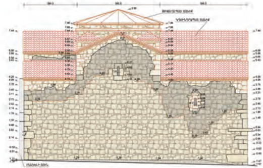
ՀՈՒՄԱՍԱՆԻ ԾԱԿԱՏ 1:50
