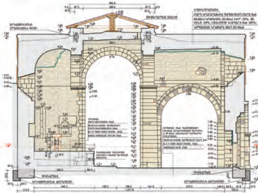
ԿՏՐԱԿԱՆ ԿԵՆՏՐՈՆԻ ԴԵՊԻ ՀԱՐԿԱՆ 1:50
