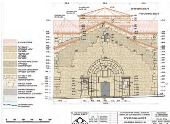
ԿՏՐԱԿԱՆ ԿԵՆՏՐՈՆԻ ԴԵՊԻ ԱՐԵՎԱՏԻՔ 1:50
