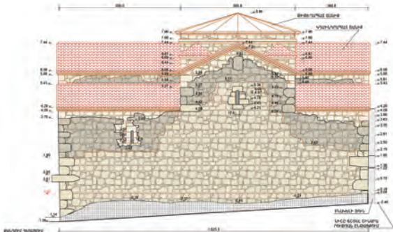
ՀԱՐԿԱԿԱՆ ԾԱԿԱՏ 1:50
