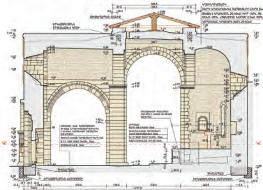
ԿՏՐԱԿԱՆ ԿԵՆՏՐՈՆԻ ԴԵՊԻ ՀՈՒՄԱՍ 1:50
